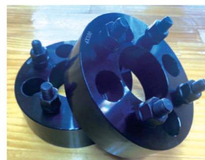
ワイドレッドスペーサーPCD100 4穴 20mm ¥9,900 30mm ¥10,450 40mm ¥11,000 50mm ¥12,100 60mm ¥13,200 70mm ¥14,300
