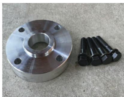
プロペラシャフトスペーサー20mm フロント ¥11,000 リア ¥11,500
